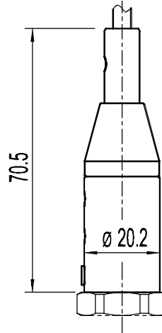
Cable outlet
