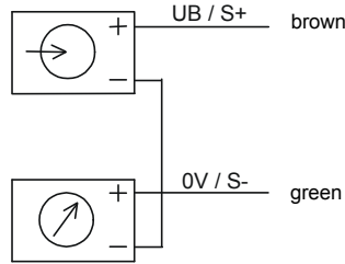
Cable outlet
